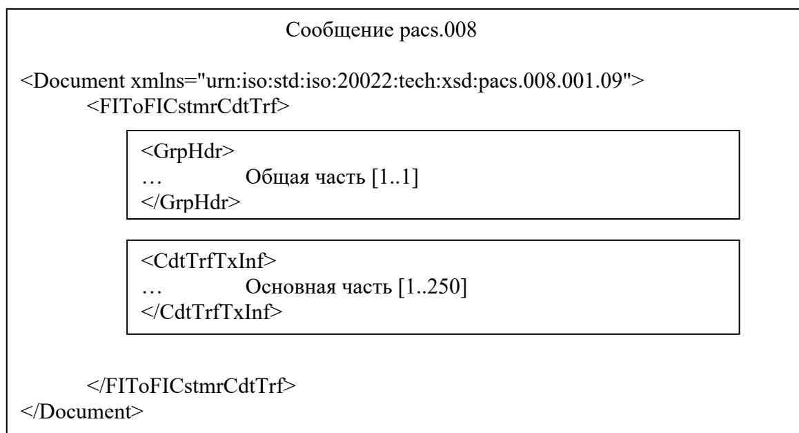
Рисунок 1 – Структура МХ-сообщения pacs.008
